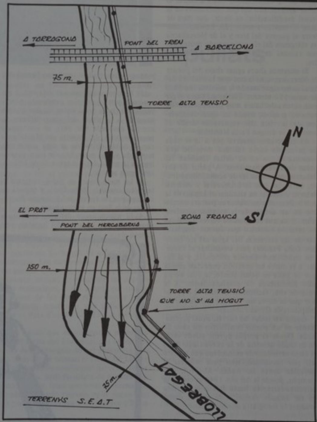
Explicació gràfica realitzada per DELTA de com incidiria la forta corrent d'una riada contra el marge d'El Prat al sector del pont de Mercabarna.
