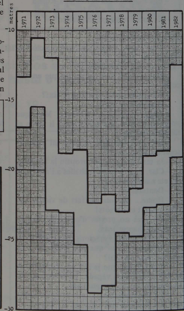
EVOLUCIO NIVELLS PIEZOMETRICS - ZONA TERLENKA
