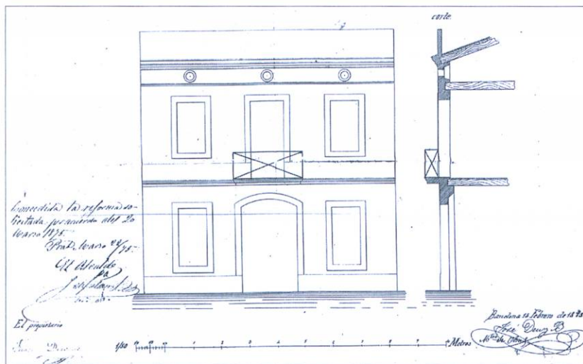
Plànol de la casa que d. Joan Deixens pretenia edificar al Prat.
